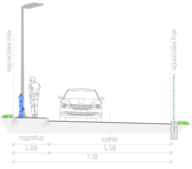
PRESJEK E
