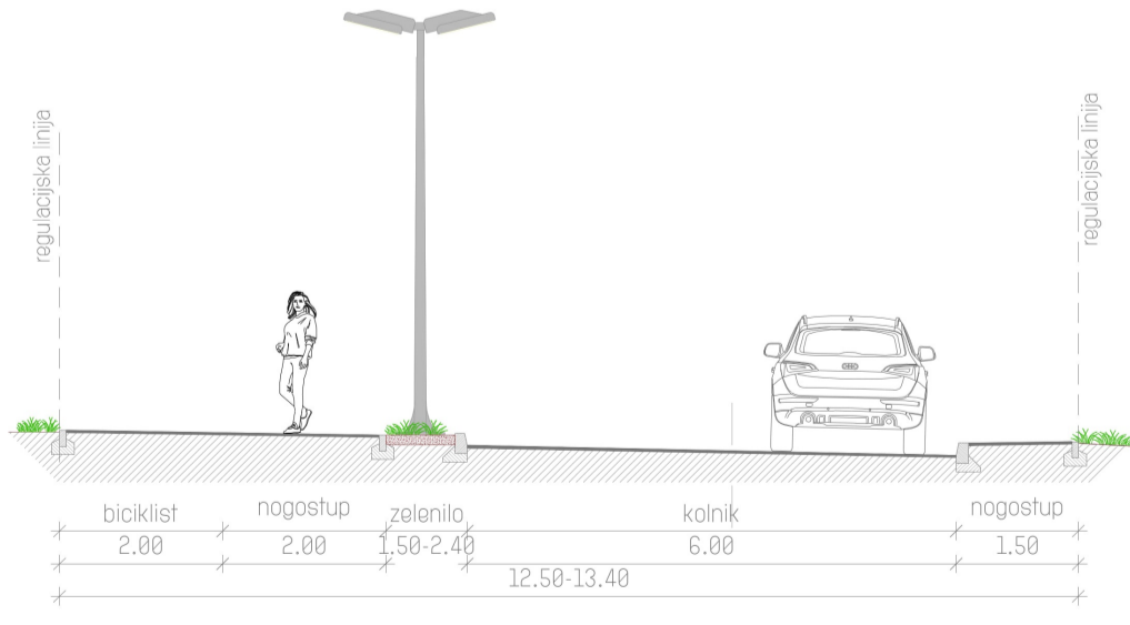
PRESJEK G biciklističke i pješačke staze
