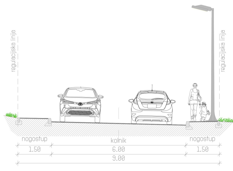
PRESJEK E
