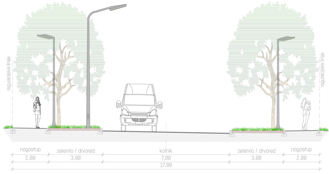
PRESJEK D
