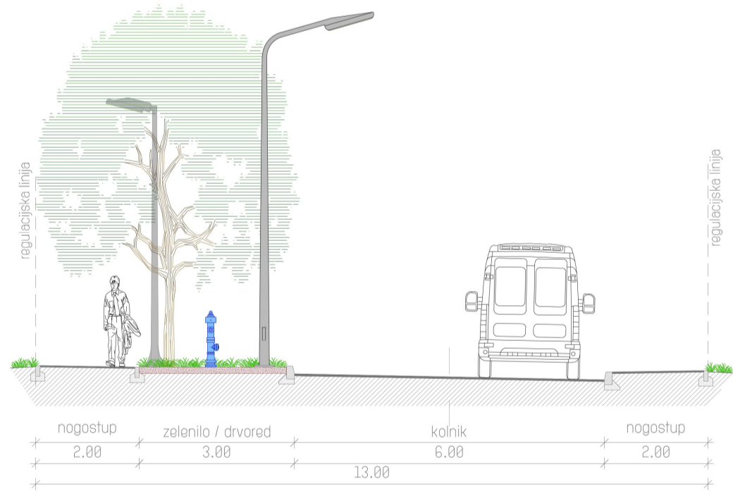
PRESJEK C
